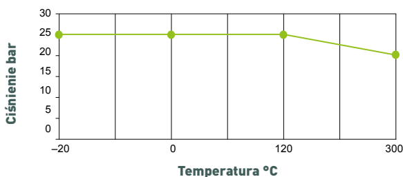
Stosunek ciśnienia i temperatury
