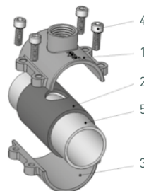
1. Górną część z odejściem w gwintem wewnętrznym 2. Uszczelka z otworem 3. Dolną część 4. Śruby 5. Rura
