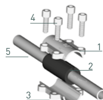
1. Górną część 2. Uszczelka 3. Dolną część 4. Śruby 5. Rura
